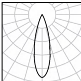
5W Ra92 3000K 24°
