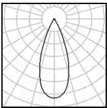
3W Ra98 3000K 46°
