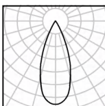
7W GREEN 36°
