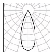
8W Ra92 3000K 36°
