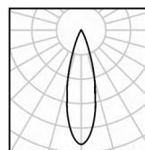
8W Ra92 3000K 24°
