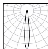
8W Ra92 3000K 15°
