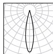
8W Ra98 3000K 28°
